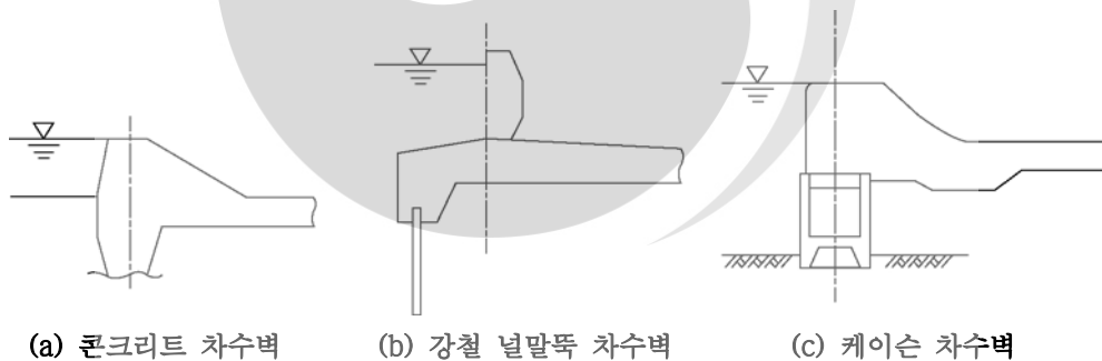
그림 4.4-1 차수벽의 종류
