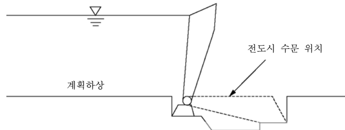
그림 4.3-2 개량식보의 형상
