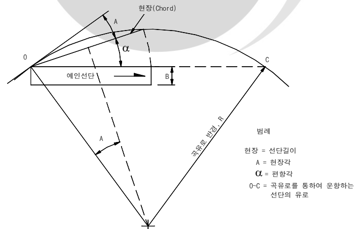
그림 4.2-1 만곡수로에서의 편향각
