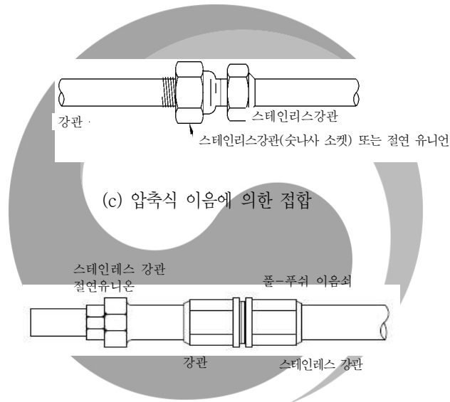
(d) 물-푸쉬이음(SU 조인트)에 의한 접합
