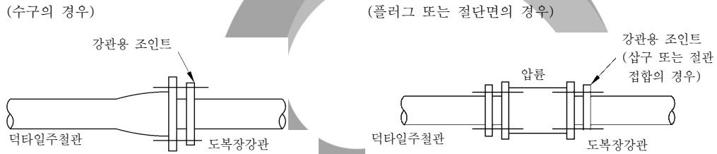
(c) 접분에 의한 접합
