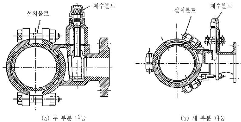
그림 2.2-2 부단수분기 정자관
