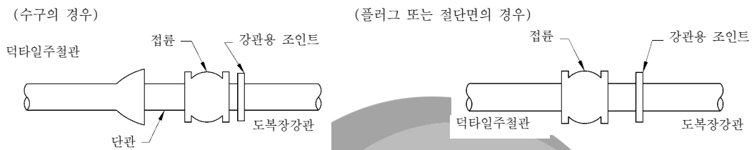
(b) 이음부속에 의한 접합
