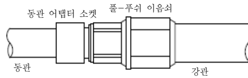
(d) 플-푸쉬이음(SU 조인트)에 의한 접합
