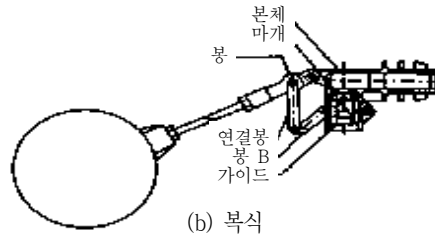
그림 3.7-2 볼밸브
