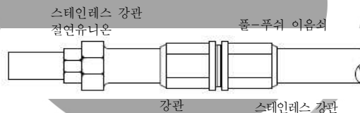
(d) 물-푸쉬이음(SU 조인트)에 의한 접합
