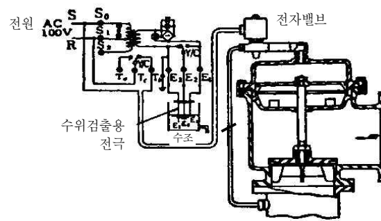
(b) 전자밸브
