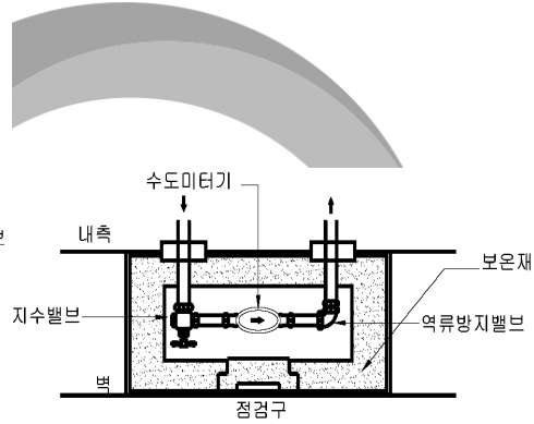
(c) 공동주택 벽 보호함(평면도)
