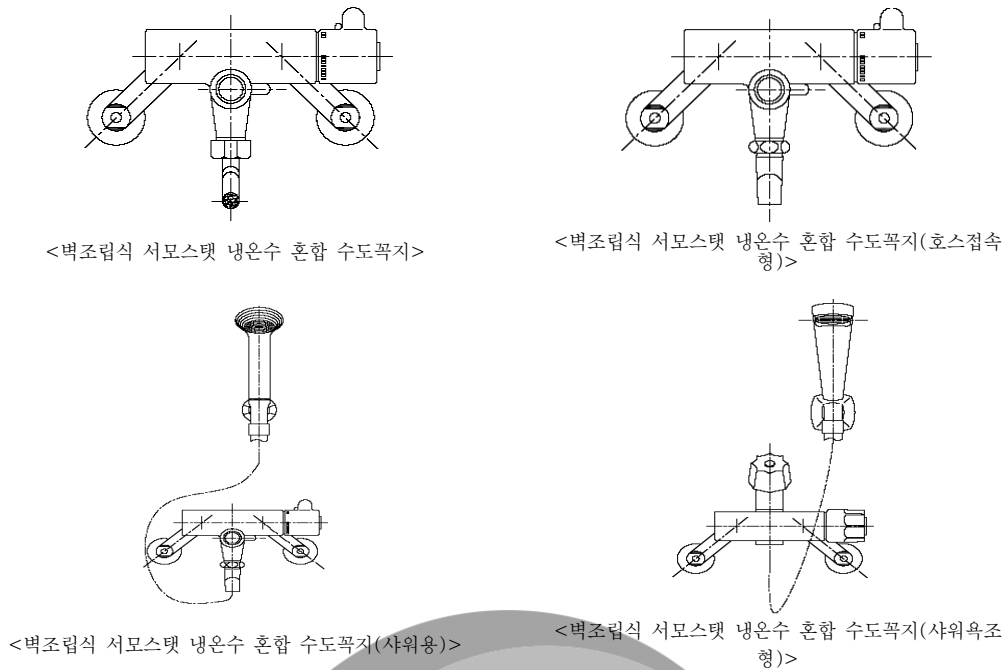
그림 3.7-1 수도꼭지
