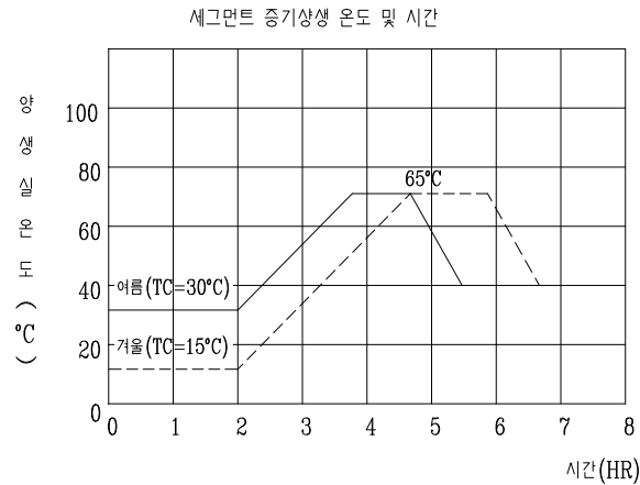
그림 3.4-2 세그먼트 증기양생 온도 및 시간
