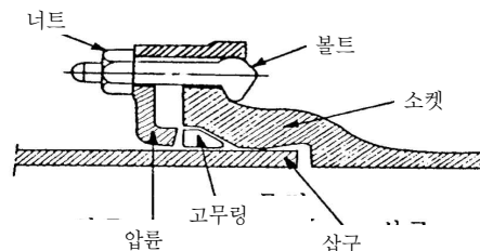
그림 3.1-2 KP메커니컬접합의 이음구조
