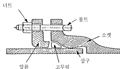
그림 3.1-1 메커니컬접합의 이음구조
