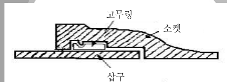
그림 3.1-3 타이튼접합의 이음구조
