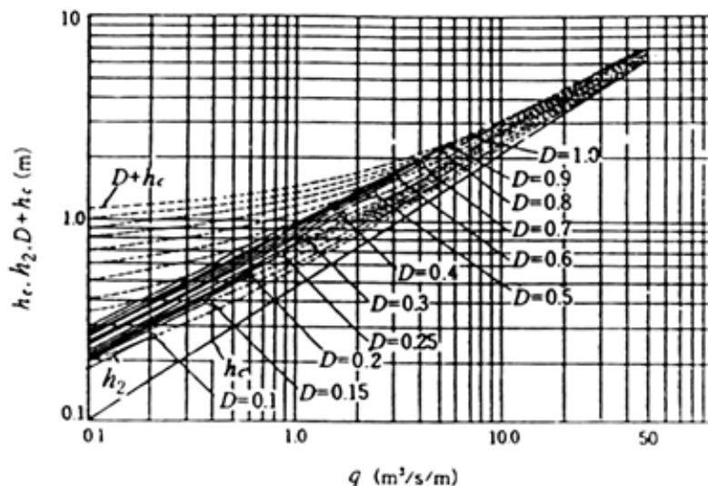
<그림 1.2-1> 보 하류의 유수영역 판정 도표 ( D=0.1\sim 1.0\text{m} )
