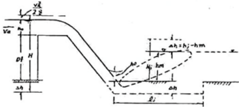
〈그림 1.8-1〉 물방석
