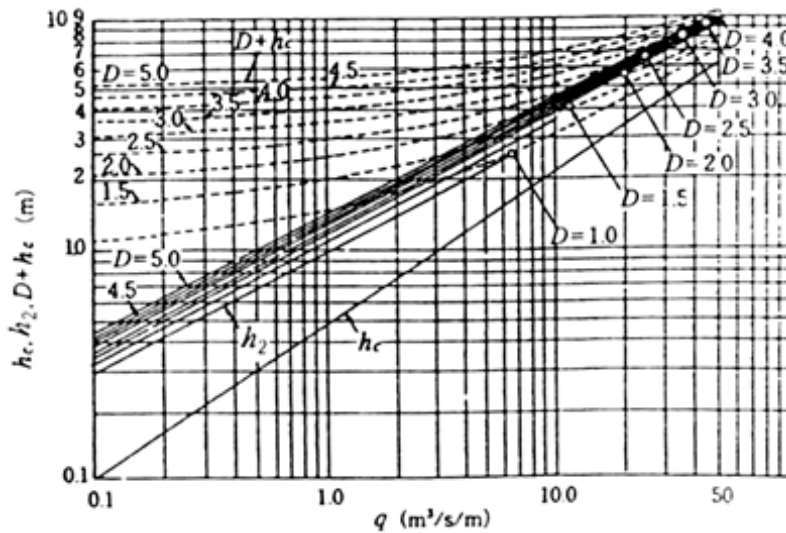
〈그림 1.2-2〉 보 하류의 유수영역 판정 도표 ( D=1.0\sim4.0\text{m} )
