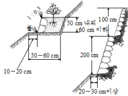
〈그림 2.4-4〉 석축공
