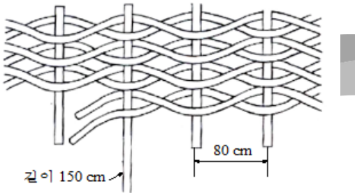
〈그림 2.4-5〉 편책공
