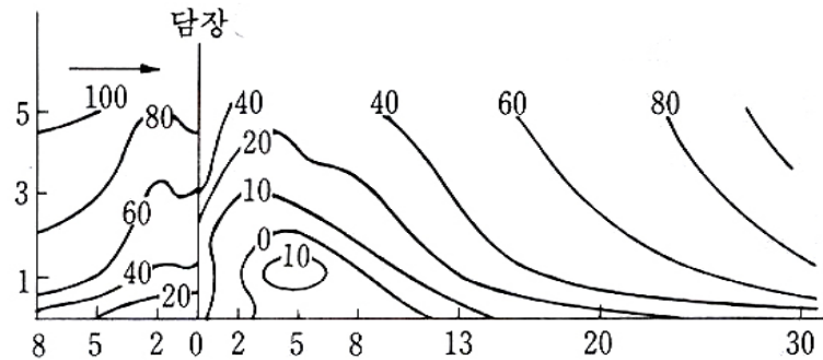
<그림 2.4-1> 방풍담장 부근의 비풍속 분포도
