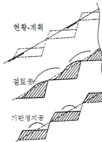
〈그림 4.1-2〉 전단면 절토공법
