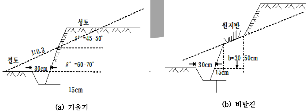
&lt;그림 4.1-4&gt; 계단 비탈면
