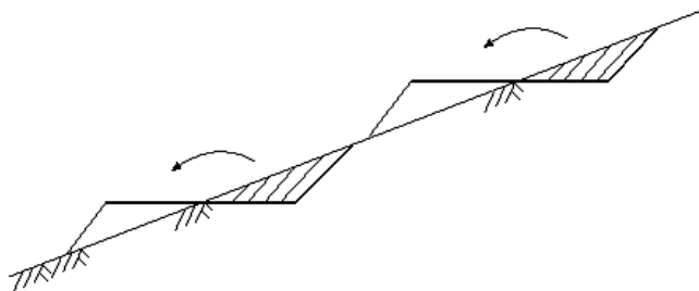
<그림 4.1-1> 절·성토공법
