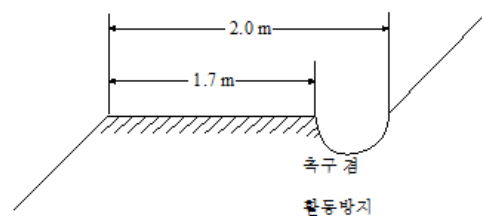
<그림 4.3-9> 경작도의 단면
