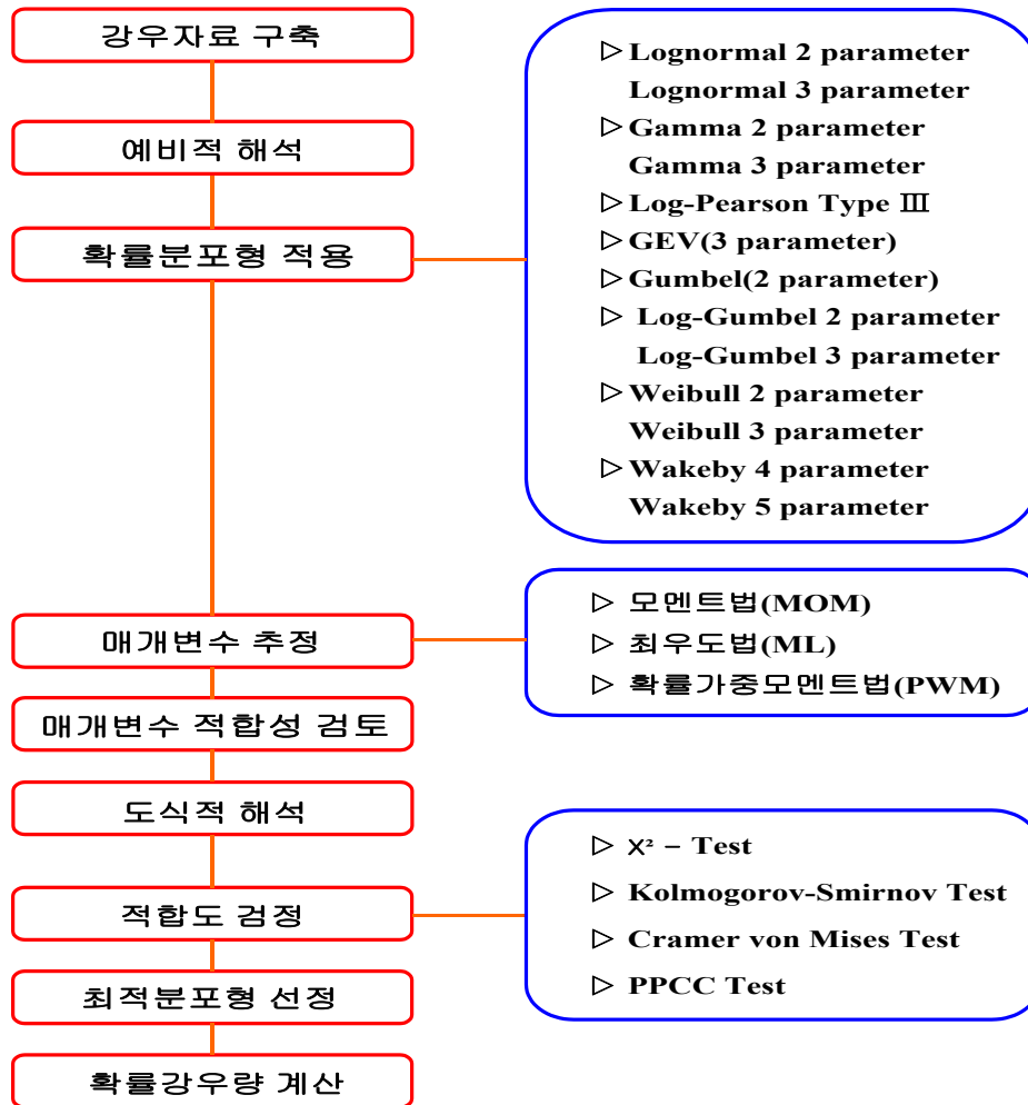
〈그림 5.1-2〉 강우빈도 해석 절차
