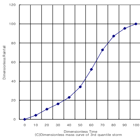
<그림 5.1-3> Huff 분포에 의한 무차원 누가곡선(금산지방)
