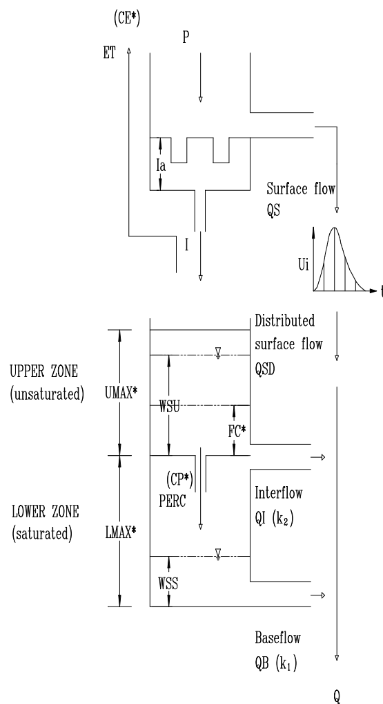
〈그림 3.2-5〉 DAWAST 모형의 개념도
