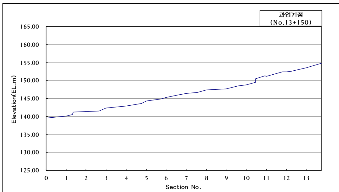
〈그림 3.3-1〉 금산천 종단 특성
