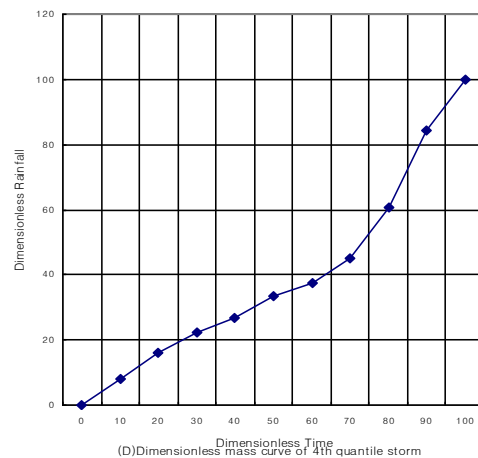
<그림 5.1-3> Huff 분포에 의한 무차원 누가곡선(금산지방)
