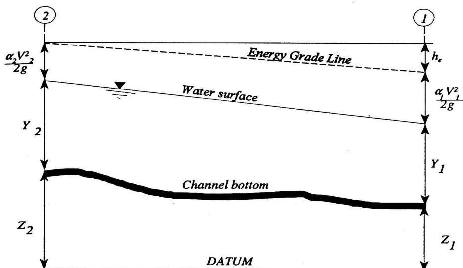
<그림 5.3-1> 표준축차계산법 모식도
