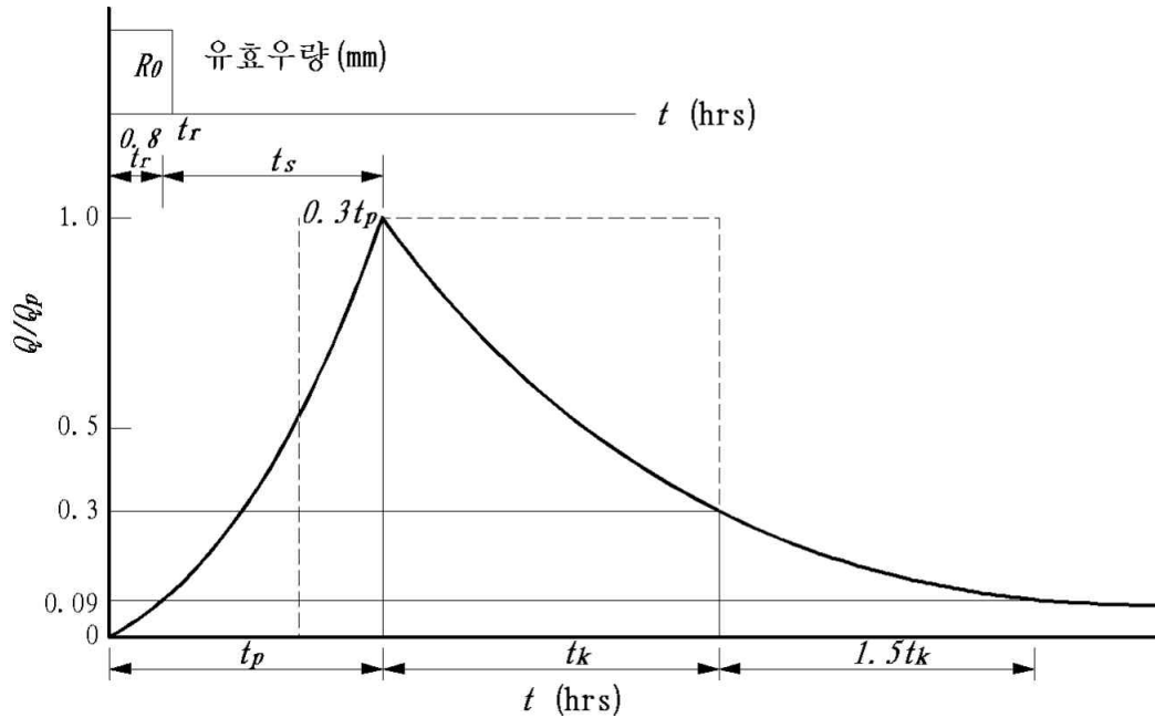
〈그림 5.1-7〉 중안(Nakayasu)의 종합단위도
