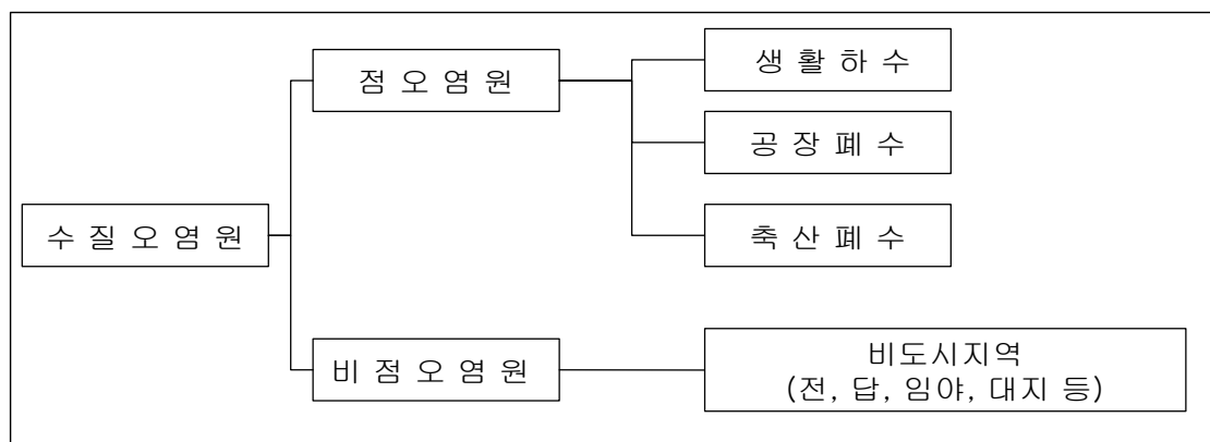
〈그림 3.6-1〉 수질오염원의 분류
