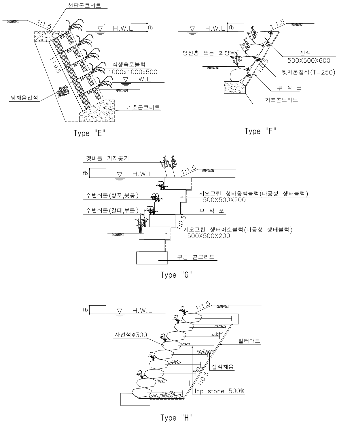
<그림 5.6-1 계속> 제방 및 호안 표준도
