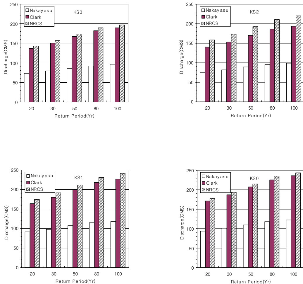
<그림 5.1-8> 지점별, 유출모형별, 빈도별 첨두홍수량 변화도
