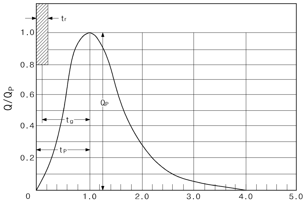
〈그림 5.1-6〉 SCS 무차원단위도
