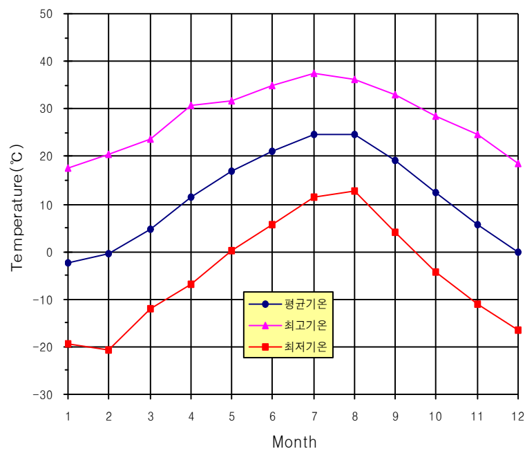
&lt;그림 3.2-1&gt; 월별 평균기온, 최고 및 최저기온 변화 추이
