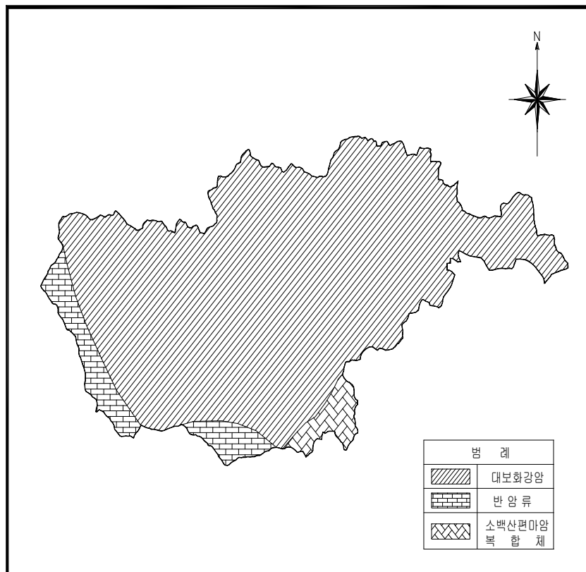
〈그림 3.1-3〉 금산천유역 지질도
