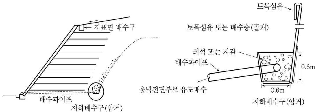
<그림 4> 보강토 비탈면의 배수시설 적용예
