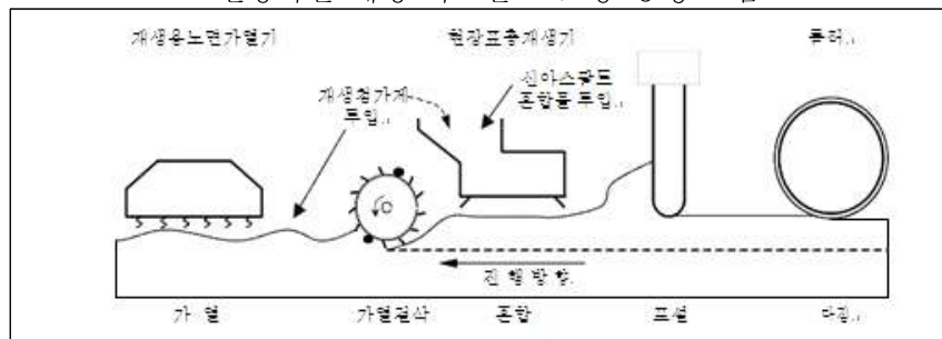
현장가열 재생 아스팔트 포장 공정 흐름
