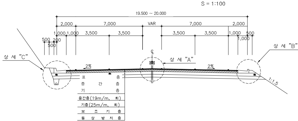
상 세 "C"
