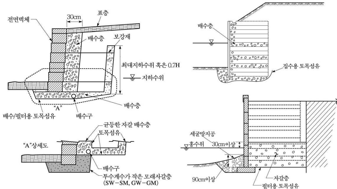
(a) 침수지역 보강토 옹벽의 배수시설
