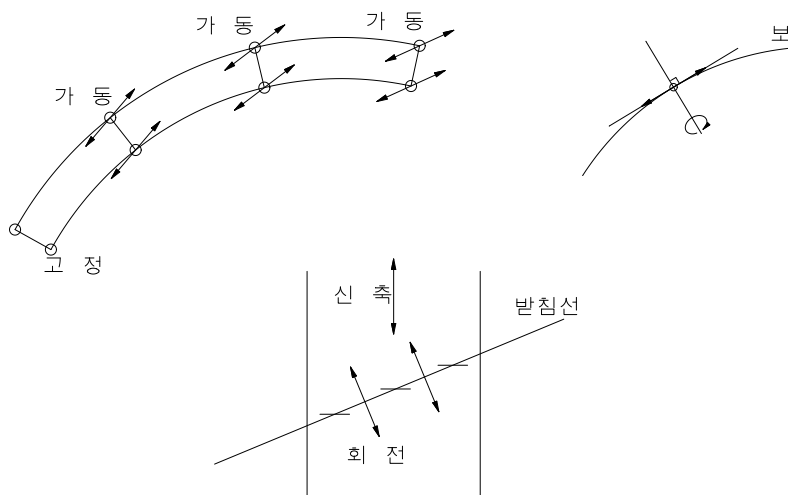
<그림1> 곡선교, 사교의 신축방향과 회전방향
