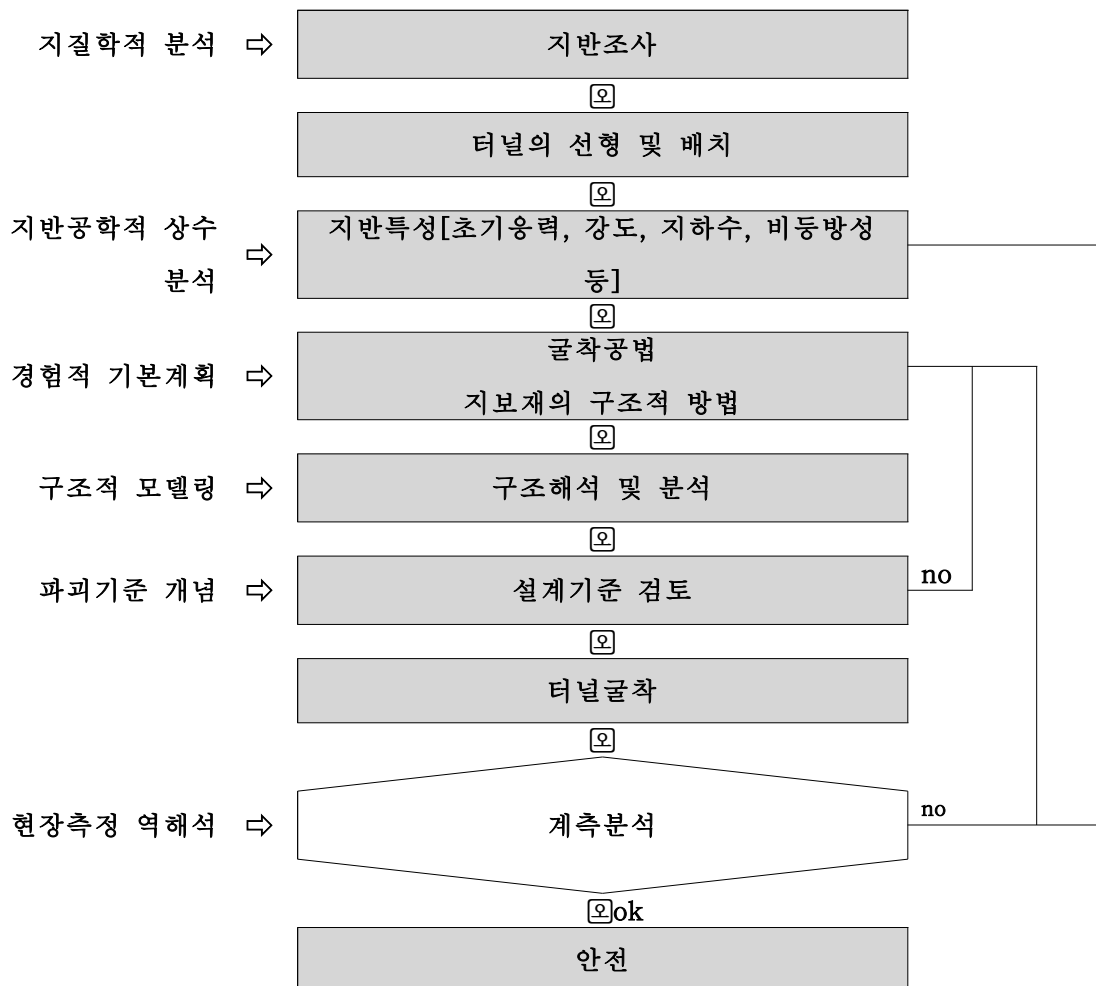
<터널설계 과정 흐름도>
