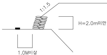
<마대쌓기>
