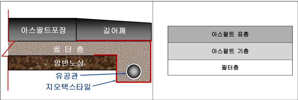
아스팔트포장의 구성
