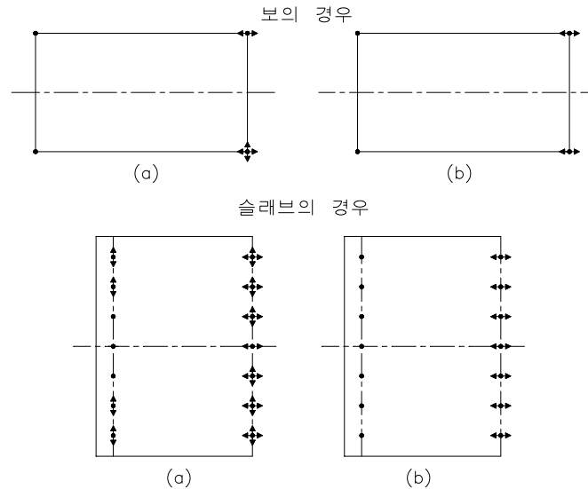
<그림2> 폭이 넓은 경우의 받침배치
