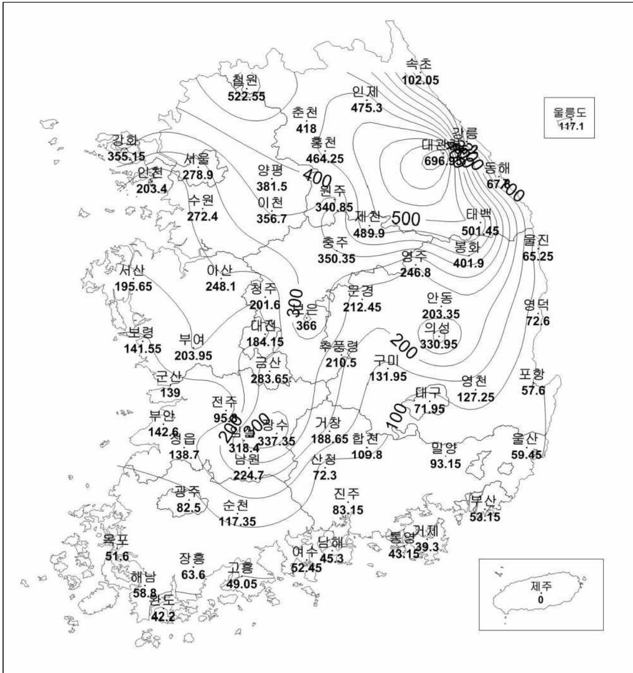
<20년 동결지수선도>
