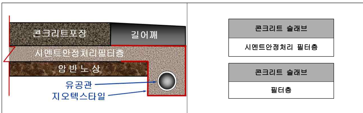
콘크리트포장의 구성
