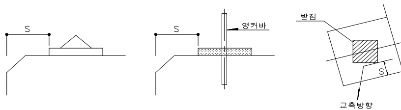
받침연단거리(S)
