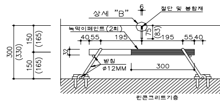
단 면 A-A
