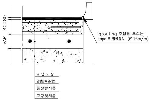
단면 A-A
