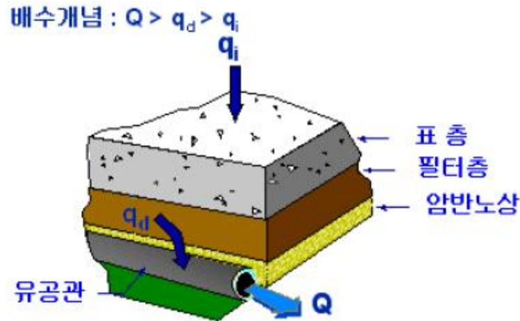
<그림 8-2> 침투수의 배수개념
