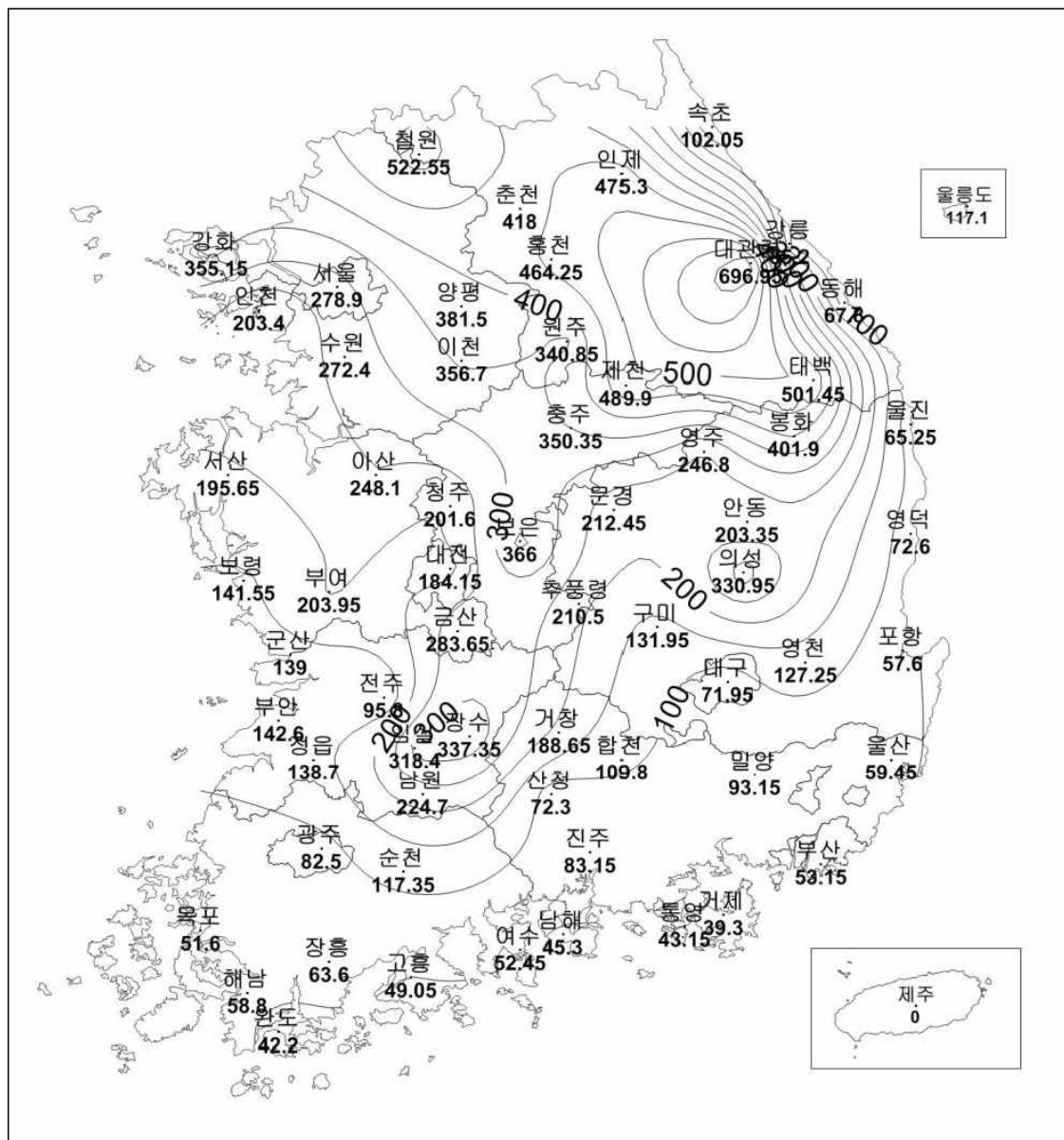
<20년 동결지수선도>
