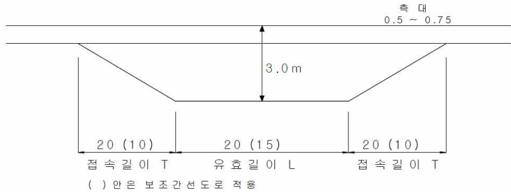
&lt; 비상주차대의 평면도 &gt;
