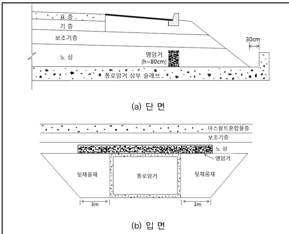
<맨암거 설치 위치>
