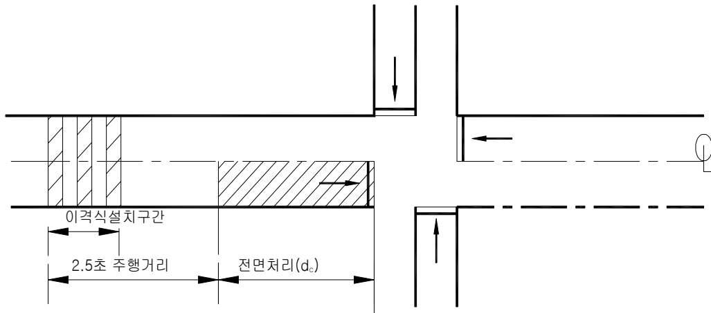
< 교차로 또는 횡단보도 접근부의 미끄럼방지 포장설치 “예” >
