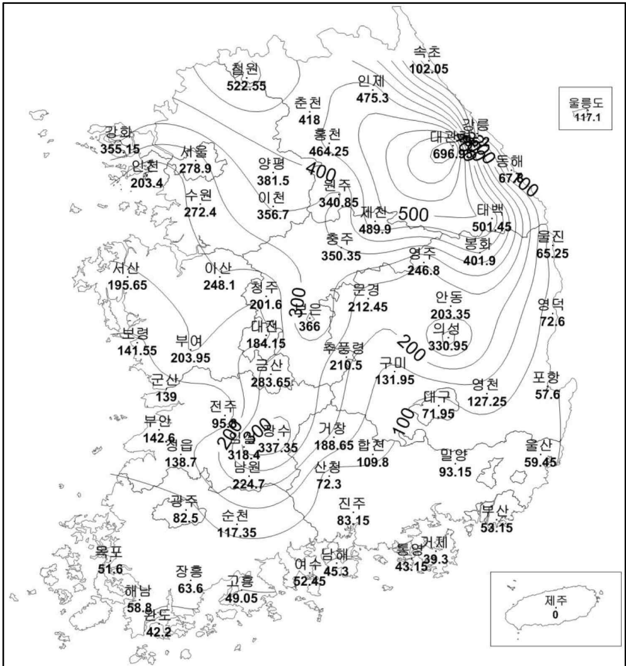
20년 전국 동결지수도
