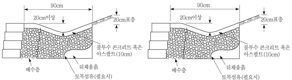
(c) 보강토 옹벽 상부 배수 및 차수대책
